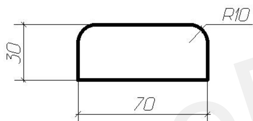
Сечение Лежня
