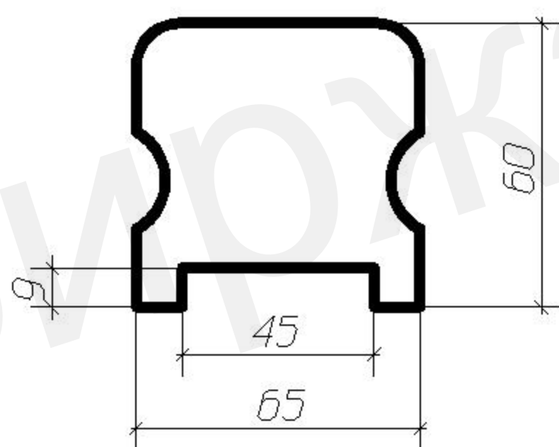
Сечение Поручня
