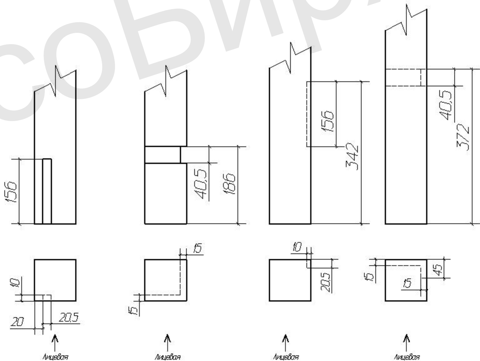
Пазы ступени, подступ Столб ограждения А
