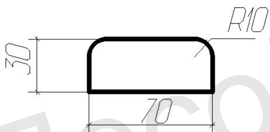
Сечение Лежня
