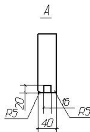
Сечение А для всех кобылок
